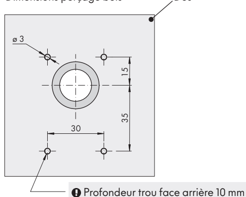
Dimensions perçage bois
